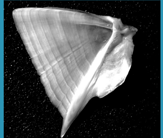
Operculum - gällocksben
